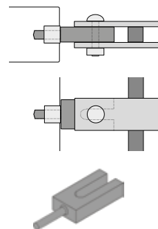
Detail uchycení plotového dílce
